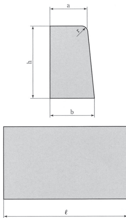
片面歩車道境界ブロック
