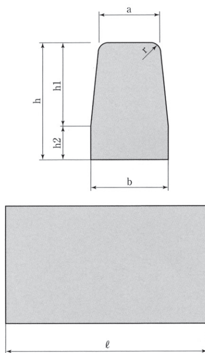
両面歩車道境界ブロック
