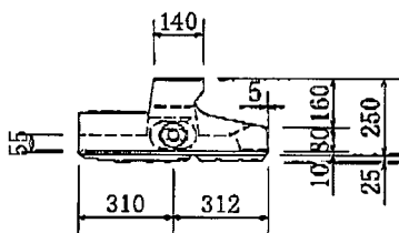
平面図
