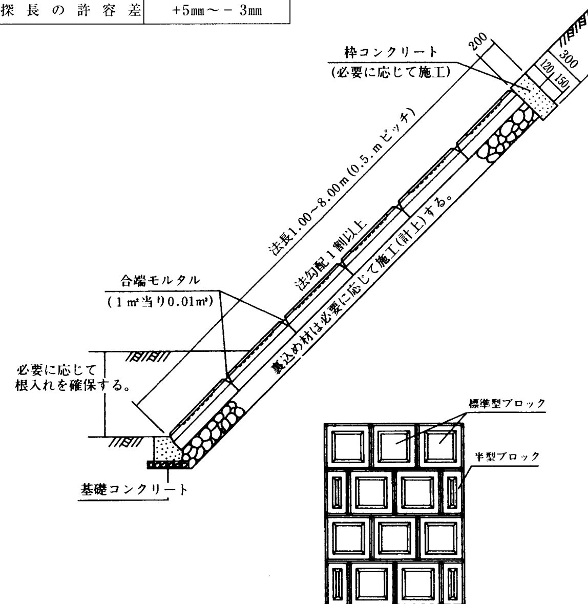
平張ブロック 1㎡当り材料表
