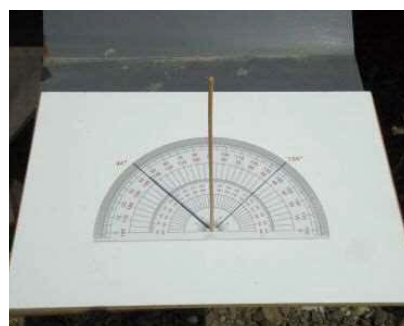
光源入射角
